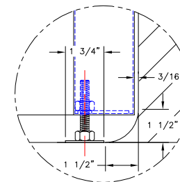
DETAIL C SCALE: 6"=1'-0"
