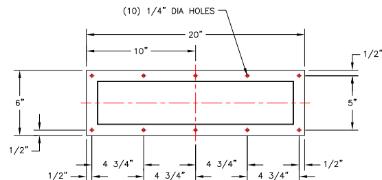
VIEW A SCALE: 3"=1'-0"
