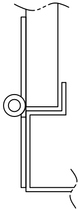
DETAIL: C-C
