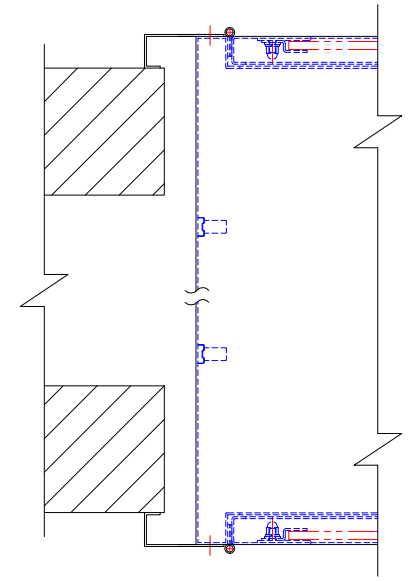
SECTION A-A SCALE: 6"=1'-0"
